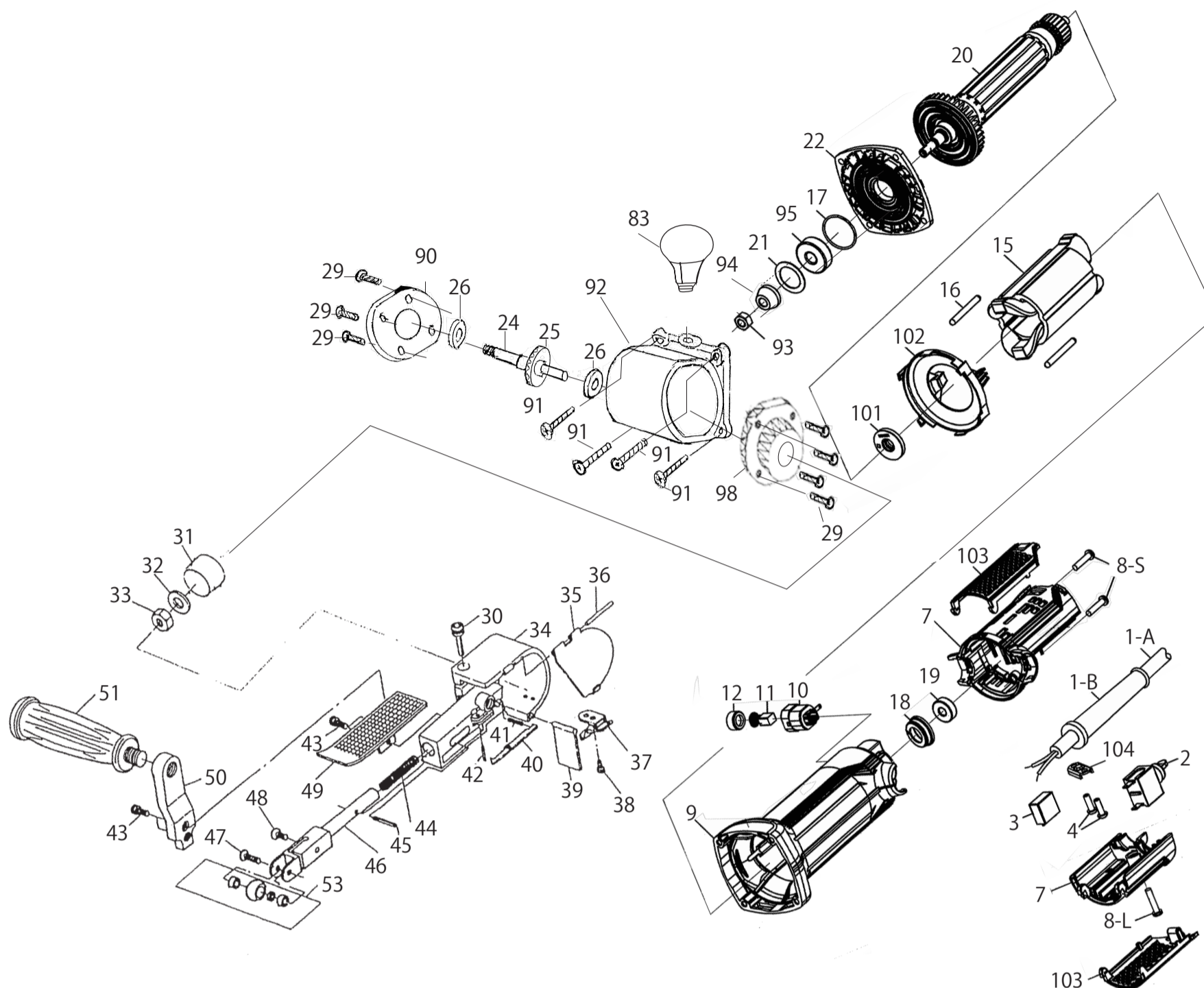
HNM-30ES 部品分解図
